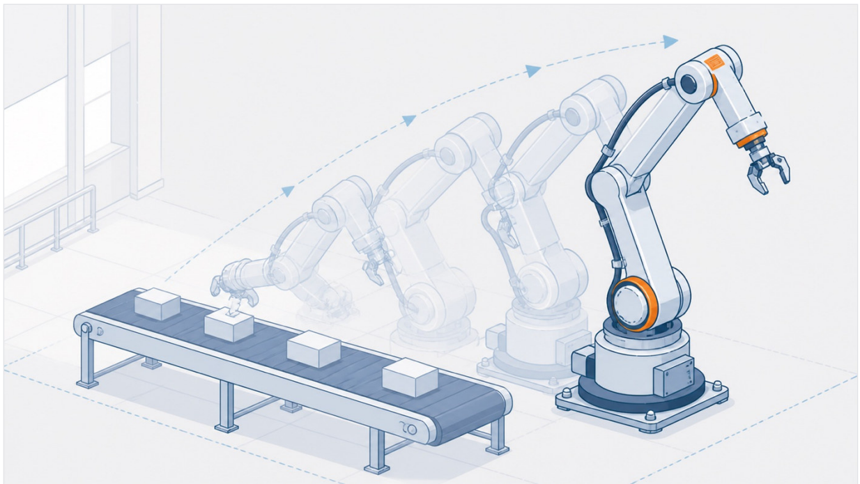
경유점 후보를 개입이 작은 순서로 시험하는 격자 탐색의 진행 — 작은 들기부터 차례로 시도한다
